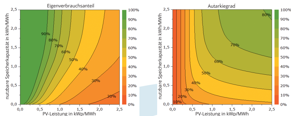
Abbildung 7: Eigenverbrauch in Abhängigkeit von Batterie- und PV-Anlagegrösse, siehe auch www.volker-quaschning.de/artikel/2013-06-Dimensionierung-PV-Speicher/index.php
