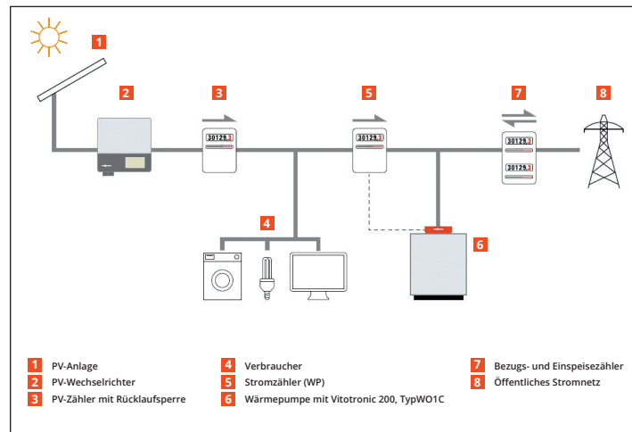
Abbildung 11: Wärmepumpen-Steuerung unter Einbezug Solarstrom von Viessmann
