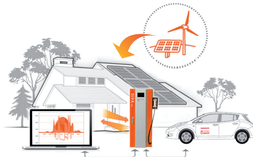
Abbildung 6: Bidirektionale Lade/Speicherstation von e8energy: Quelle: www.e8energy.de
