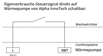
Abbildung 9 (links): Wärmepumpe an Kontakt von Wechselrichter (Quelle: ait) Abbildung 10 (rechts): Vorgesetzte Schaltvorrichtung (Quelle: Kostal)
